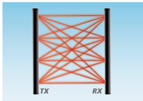
ALLINEAMENTO QUAD SMA
