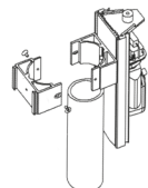
MONTAGGIO SU PALO
